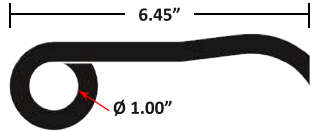
K510517232
